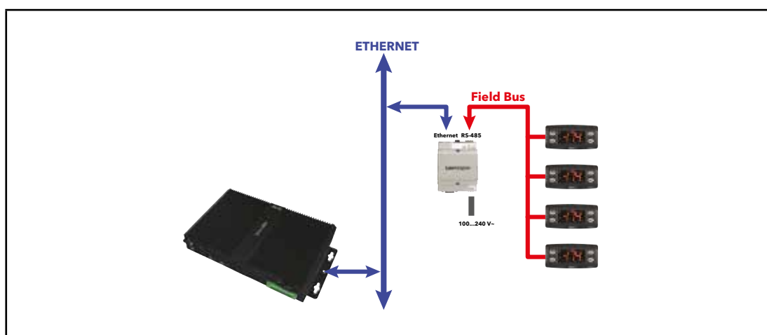
Exemple de réseau Ethernet / RS485
