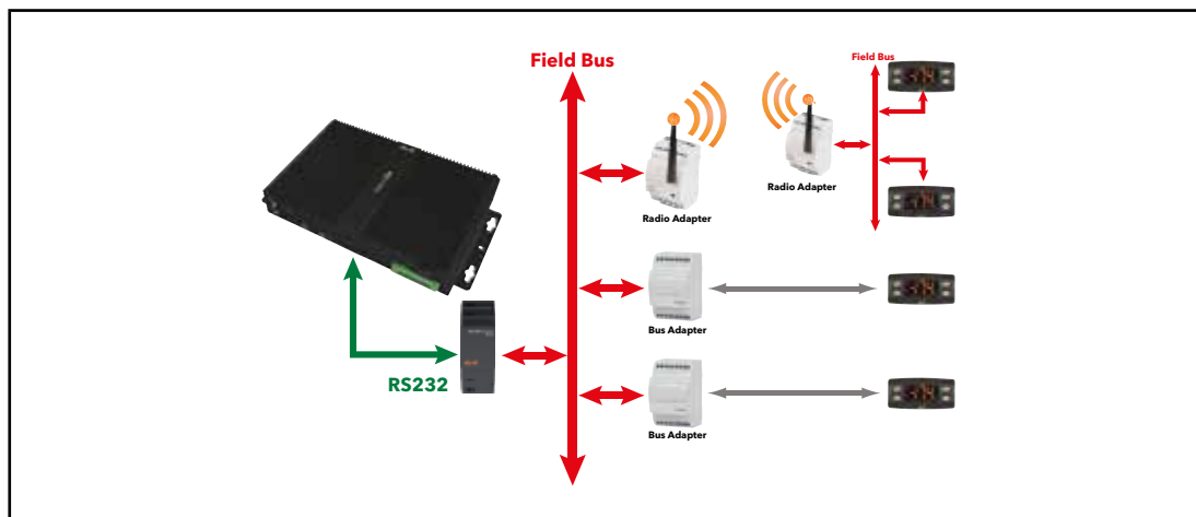
Exemple de réseau RS232 / RS485
