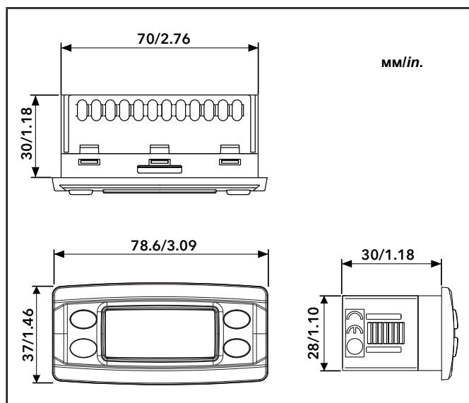
Рис. 7. Размеры
