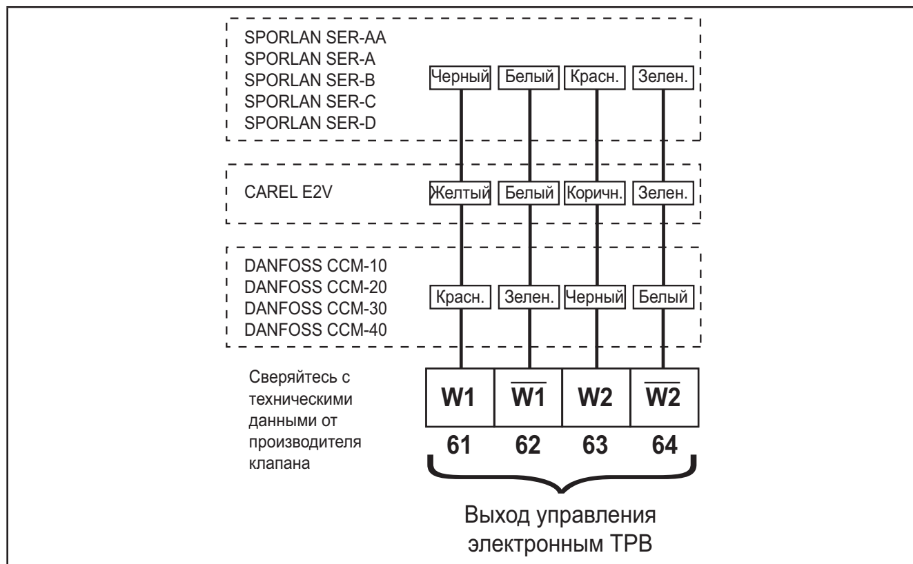
Рис. 35. Схема подключения УПРАВЛЯЕМЫХ электронных ТРВ
