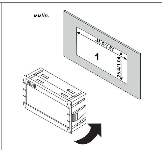
Рис. 22. Установка на панель
