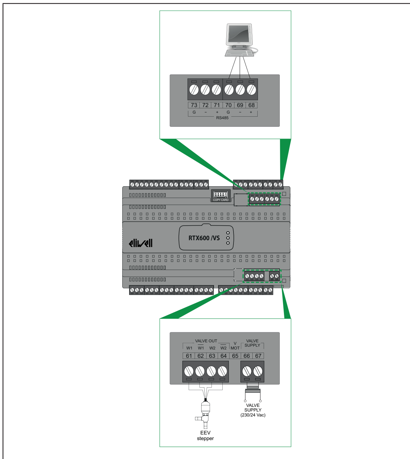
Рис. 33. Схема подключения Верхней платы
