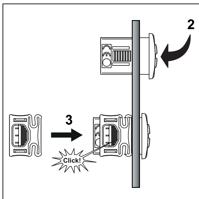
Рис. 9. Пример установки
