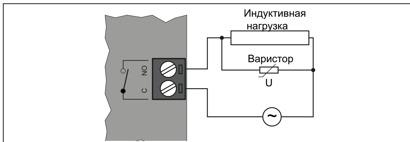
Рис. 29. Защитная цепь типа В
