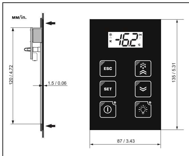
Рис. 15. Размеры
