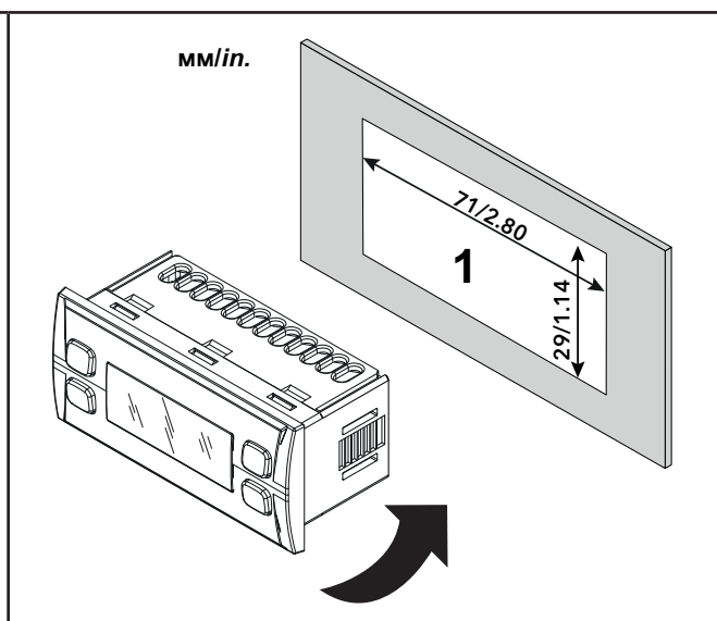
Рис. 8. Установка на панель
