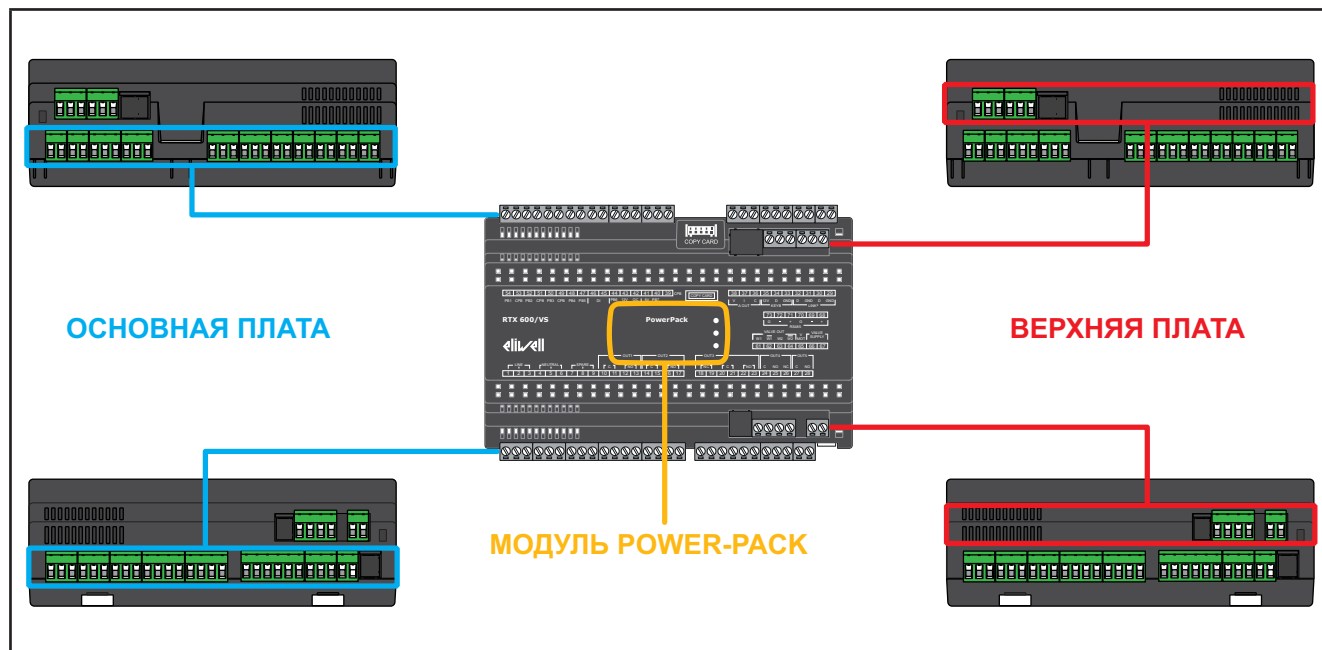
Рис. 2. RTX 600 /VS : Основная и Верхняя платы и модуль Power-Pack
