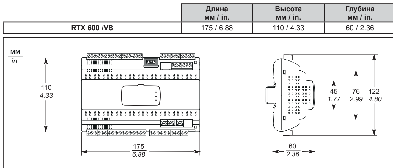
Рис. 36. Механические размеры
