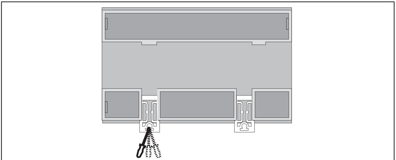
Рис. 5. Пружинная фиксация прибора
