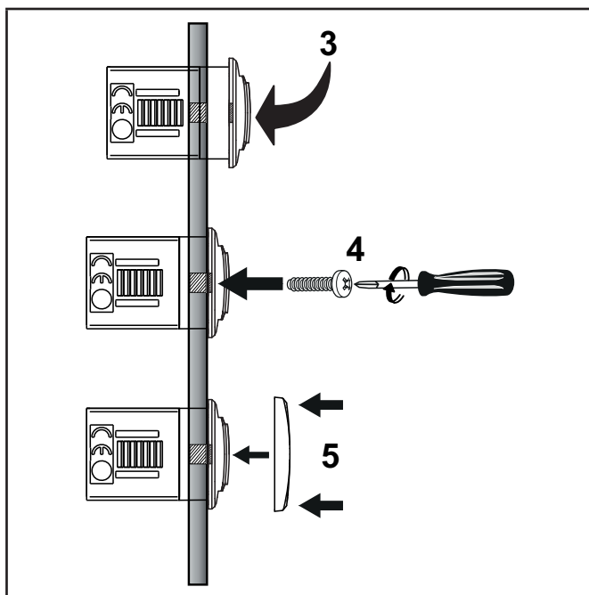
Рис. 13. Пример установки
