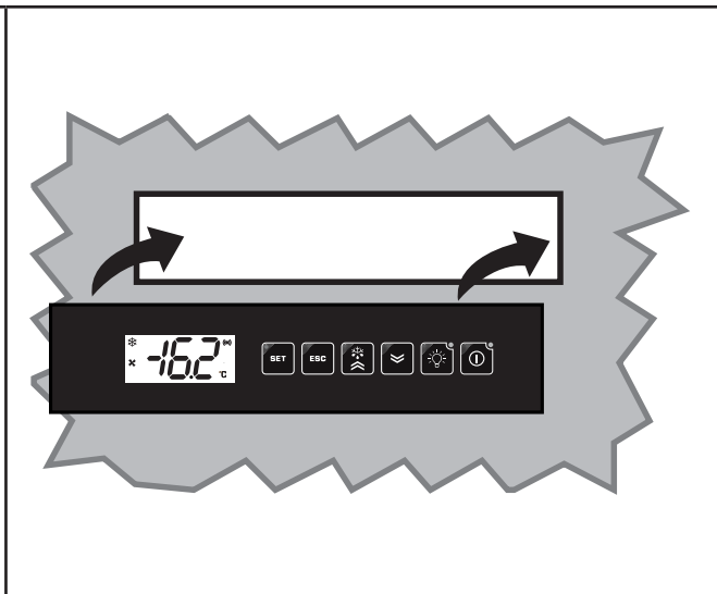
Рис. 19. Установка на панель
