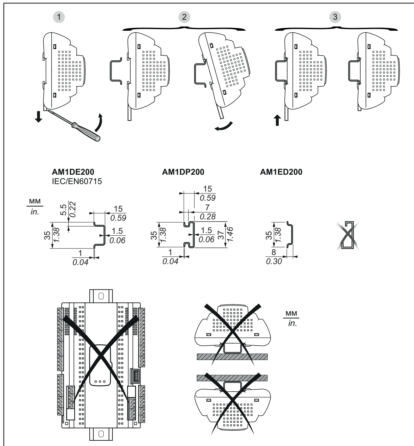
Рис. 4. Установка
