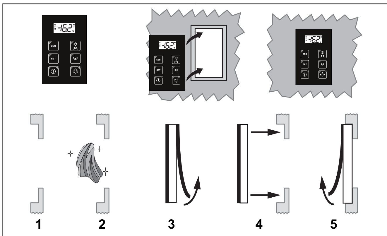
Рис. 17. Пример установки
