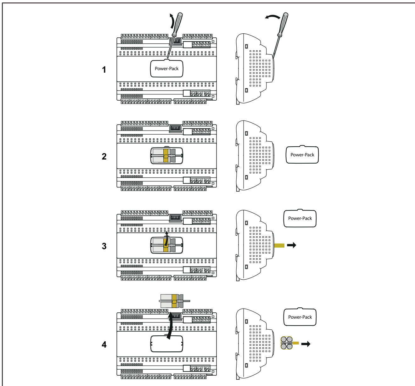
Рис. 25. Извлечение модуля Power-Pack
