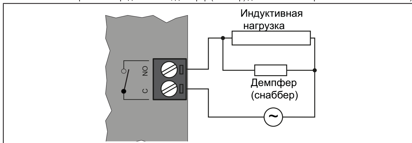
Рис. 28. Защитная цепь типа А
