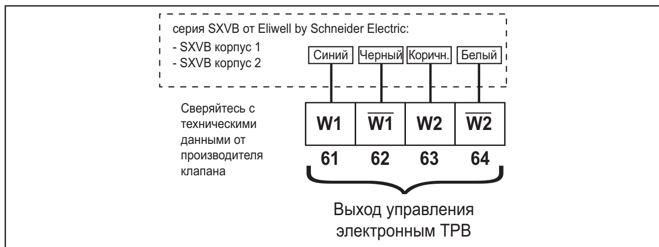
Рис. 34. Схема подключения СОВМЕСТИМЫХ электронных ТРВ
