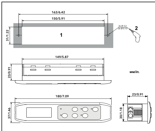
Рис. 11. Размеры
