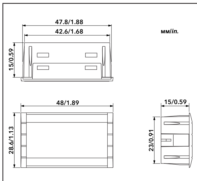
Рис. 21. Размеры
