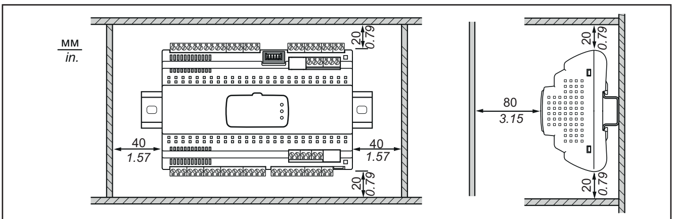
Рис. 6. Расстояния
