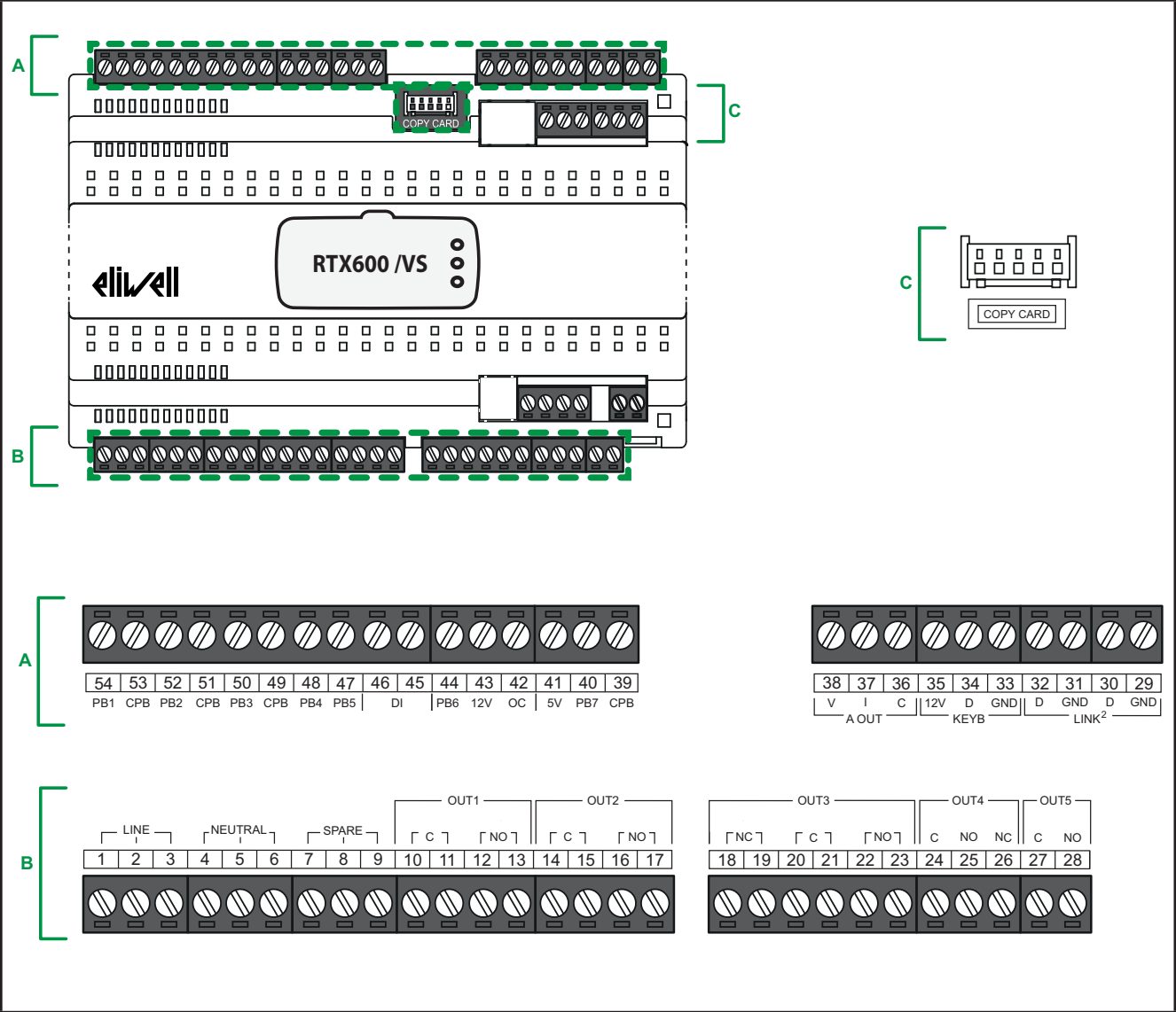
Рис. 30. Подключения Основной платы (нижний уровень)
