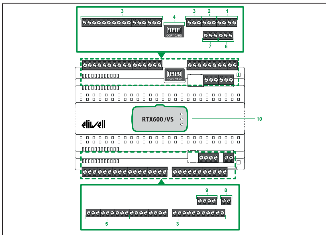
Рис. 3. Основные компоненты RTX 600 /VS
