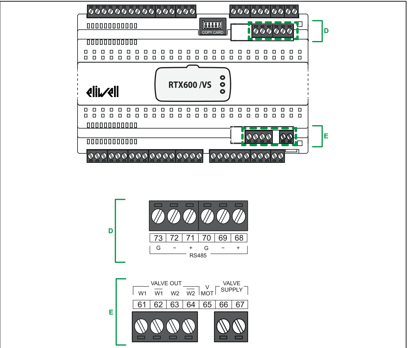
Рис. 31. Подключения Верхней платы (верхний уровень)
