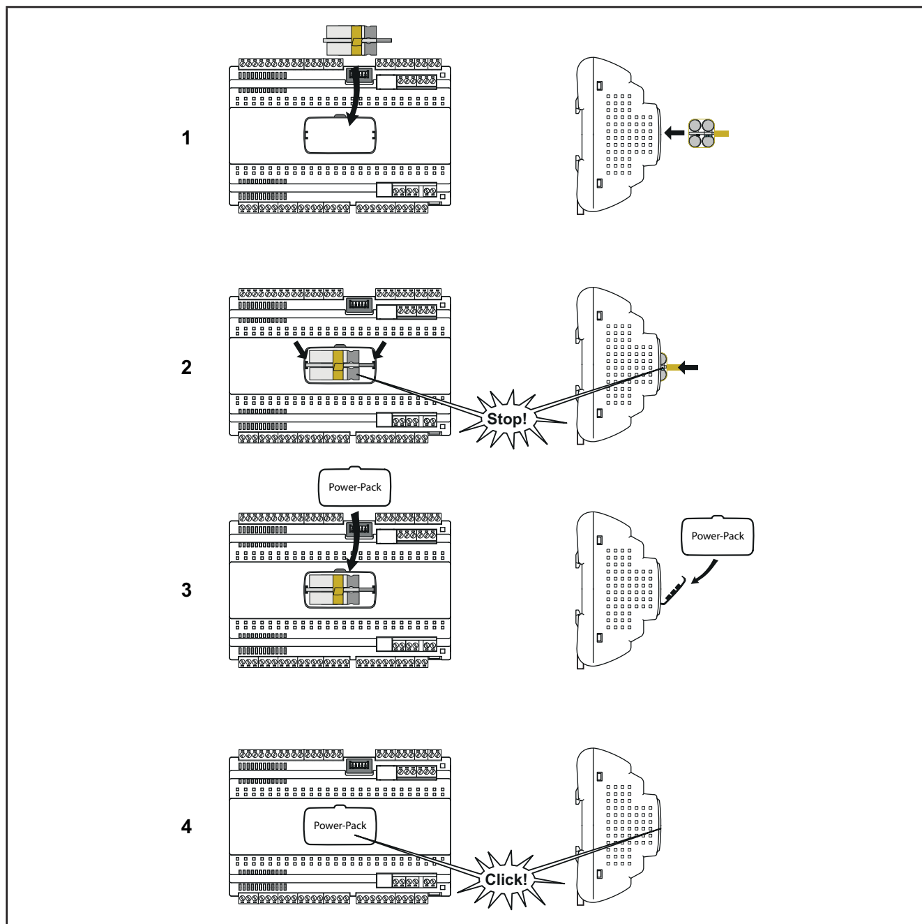
Рис. 26. Установка модуля Power-Pack
