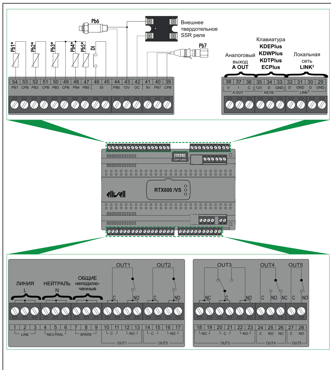
Рис. 32. Схема подключения Основной платы прибора
