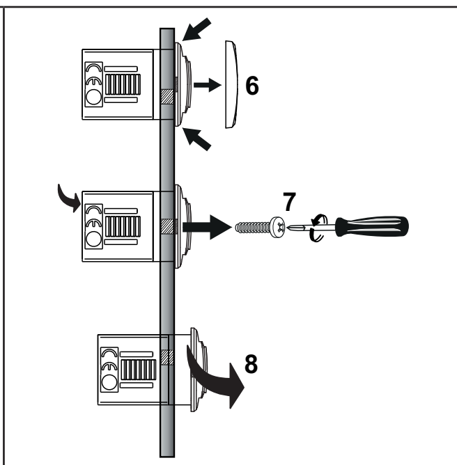
Рис. 14. Пример снятия
