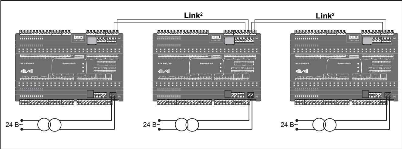
Рис. 37. Пример сети с с отдельными источниками питания электронных ТРВ
