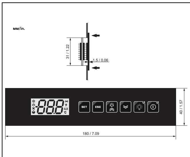
Рис. 18. Размеры
